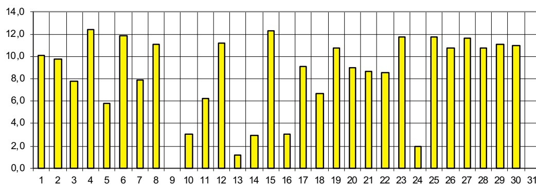
Sonnenscheinverlauf — Stunden
